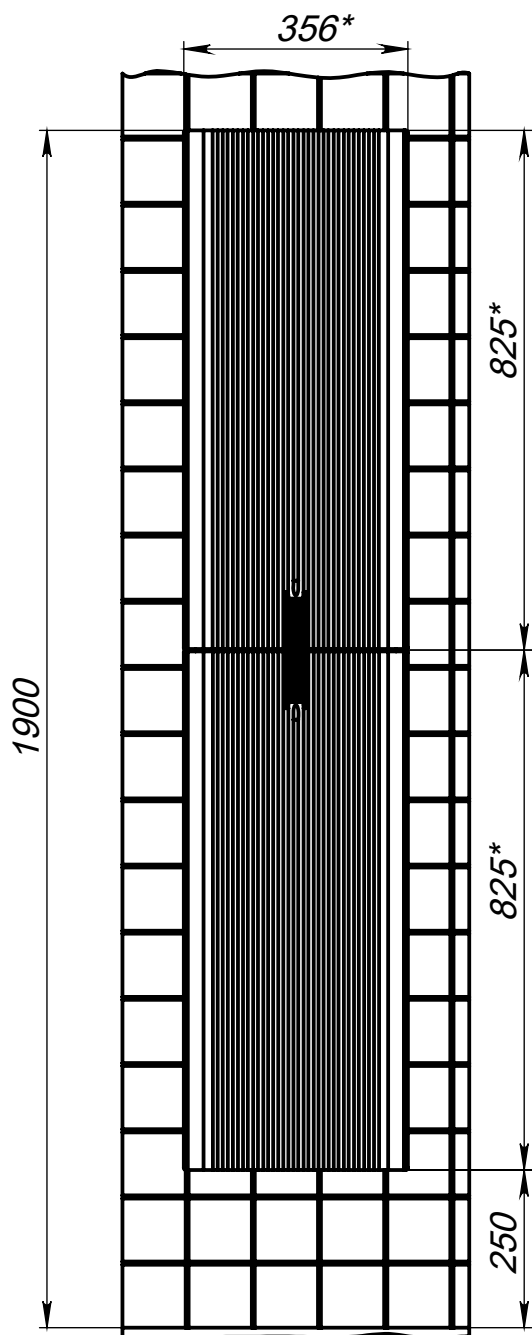
Уровень пола
